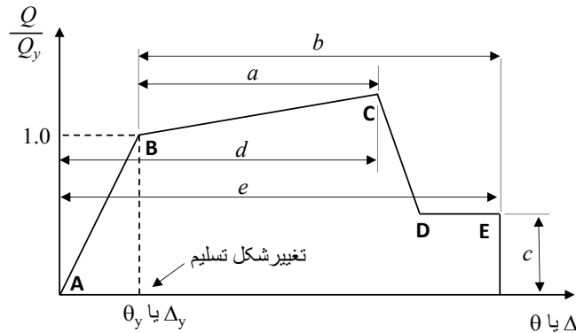
شکل پ ۱-۲ منحنی ساده شده نیرو-تغییرشکل اعضا
