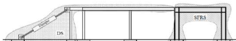
سامانه ميراگر (DS) قرار گرفته در خارج از سيستم باربر لرزه اي سازه اي (SFRS)
