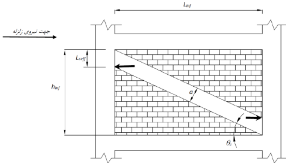
شکل پ-۲ نیروی وارد به ستون از طرف میانقاب
