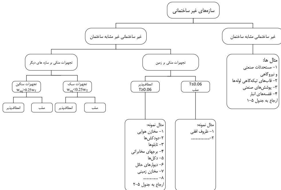
شکل پ ۸-۱ دسته بندی سازه های غیر ساختمانی
