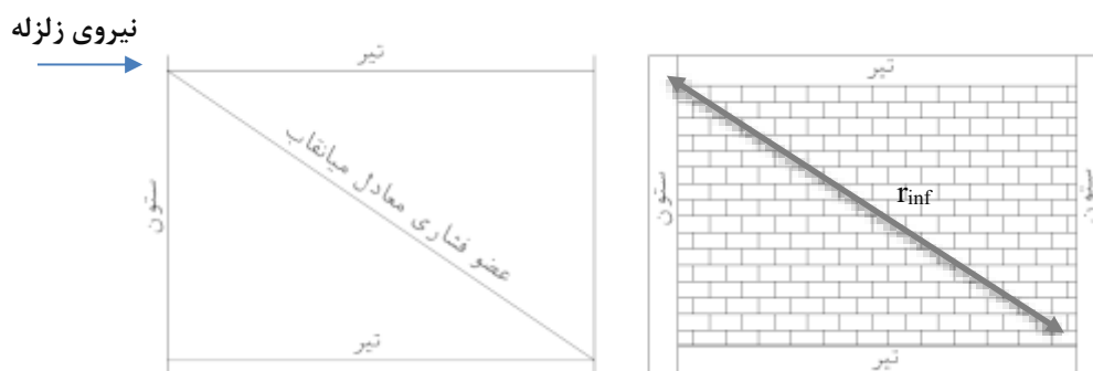
ب) مدل قاب دارای میانقاب
