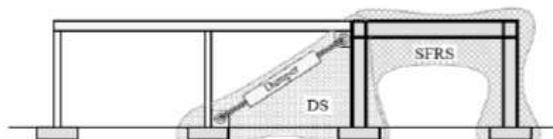
سامانه ميراگر در داخل سيستم سازه اي با برخي اعضا مشترك با سيستم باربر لرزه اي سازه
