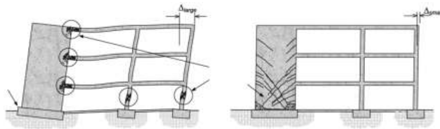
تکیه‌گاه انعطاف‌پذیر
