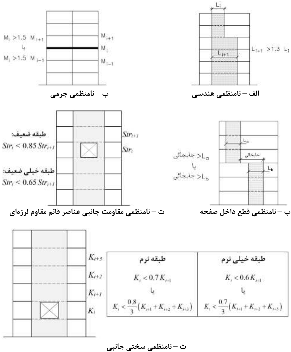
شکل ۲-۳ انواع نامنظمی در ارتفاع
