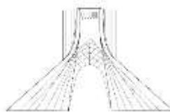
یادبودها R_{ii} = 2.5
